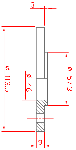
Sección A-A
